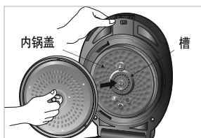
安装在锅盖时把分离式内锅盖向箭头方向对准安装槽后用力推进即可安装。
